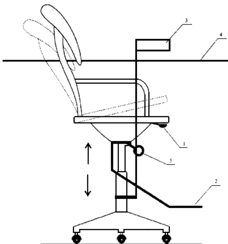
Рисунок В.12 - Трансформируемый рабочий стол для инвалида
